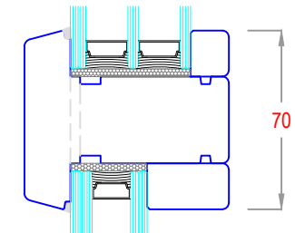
Sez. FF
