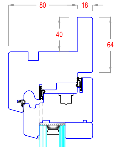
Sez. BB
