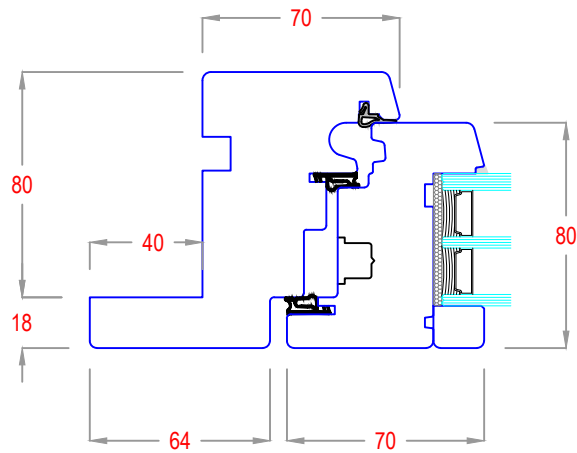
Sez. AA
