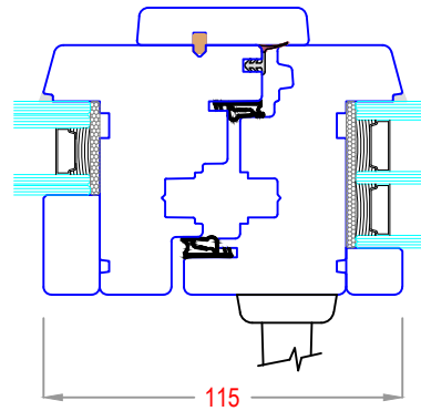
Sez. EE
